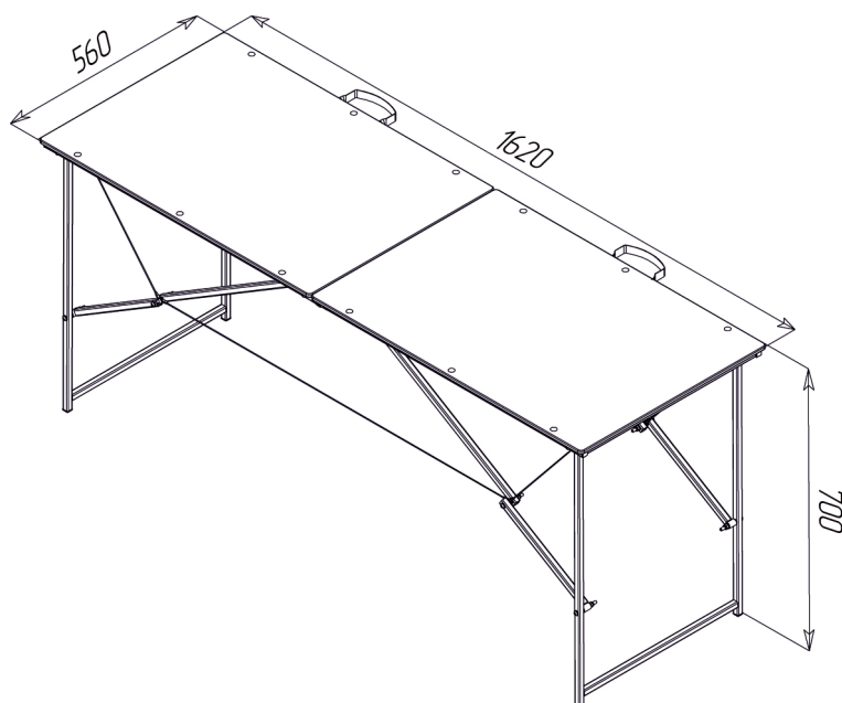
Рисунок 2 — Полок в рабочем положении
