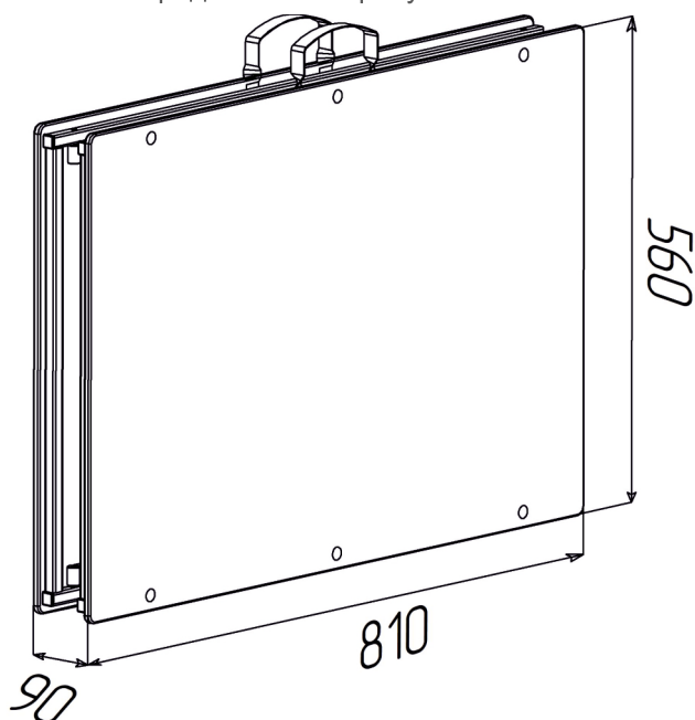
Рисунок 1 — Полок в транспортировочном положении
